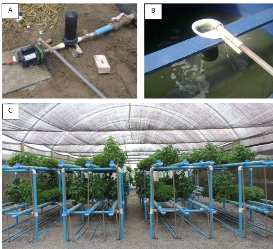
Figura 10. Filtro de tela (A), filtro de malha artesanal (B) e visão geral do experimento (C) utilizando efluente doméstico tratado em genótipos de manjerição em sistema hidropônico (ALVES, 2017).
