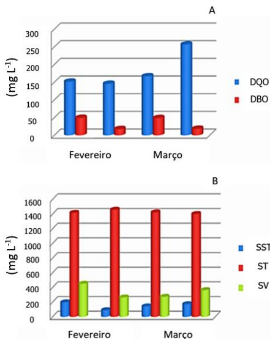
Figura 3. Comportamento das variáveis: demanda química de oxigênio (DQO), demanda bioquímica de oxigênio (DBO), sólidos solúveis totais (SST) e sólidos totais (ST) e sólidos voláteis (SV) em efluente doméstico tratado em diferentes épocas (ZAIDAN, 2010).
